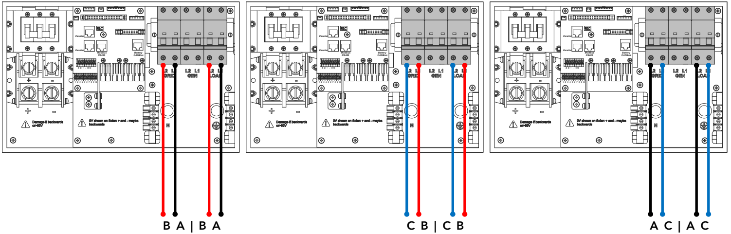
Figura 38: Ejemplo de secuencia de fases correcta
