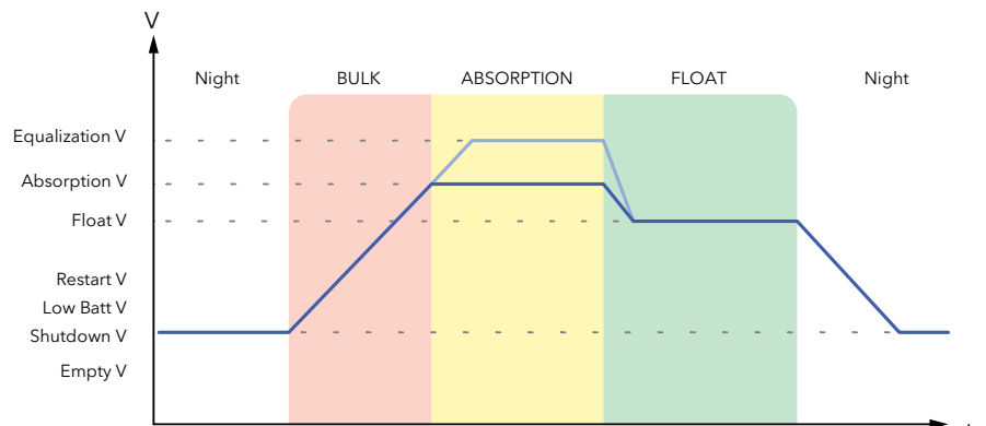
Figura 32: Curva de controlador de carga
