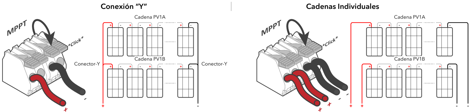
Figura 9: Cableado de MPPT y conexión de cadenas FV
