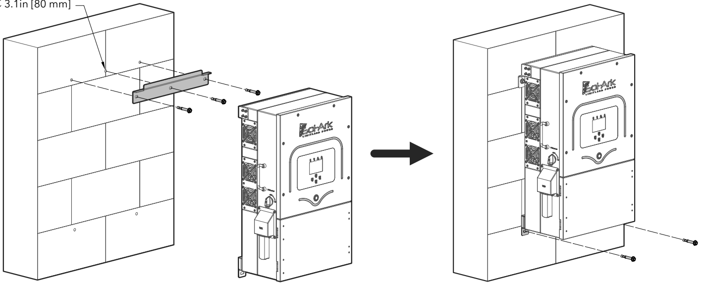
Figura 3: Montaje mural
